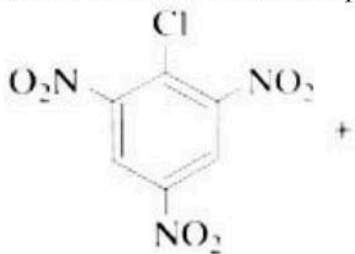
1-Chloro-2, 4, 6-trinitrobenzene
