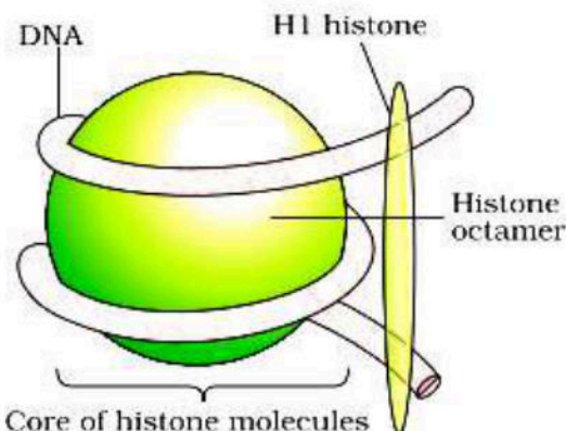
Fig: Nucleosome
